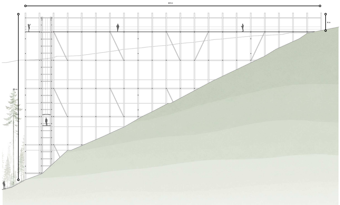
SECCION DE PLANTA E:1/320
